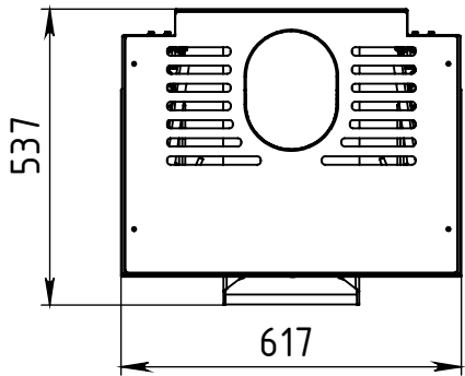
СЕЧЕНИЕ С-С
