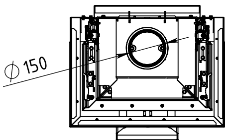
СЕЧЕНИЕ С-С
