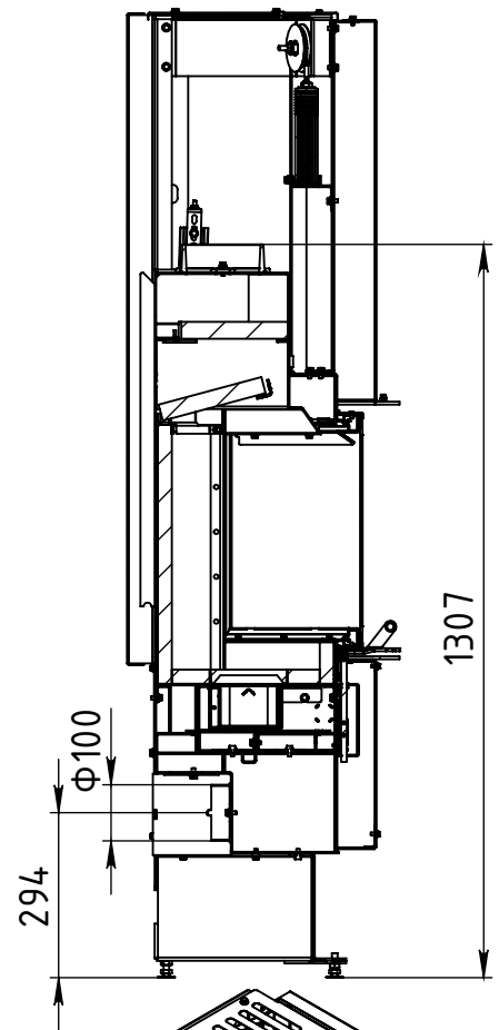
СЕЧЕНИЕ D-D
