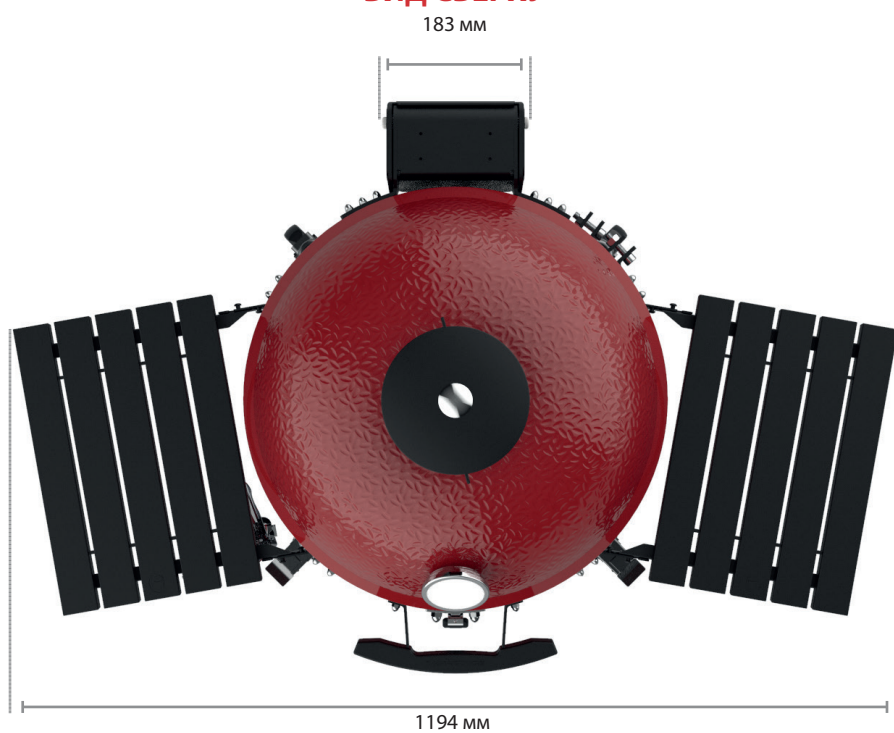
ВИД СВЕРХУ
