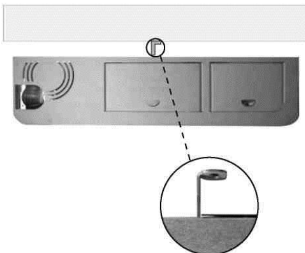
Установка розетка и fixing кронштейн на стену
